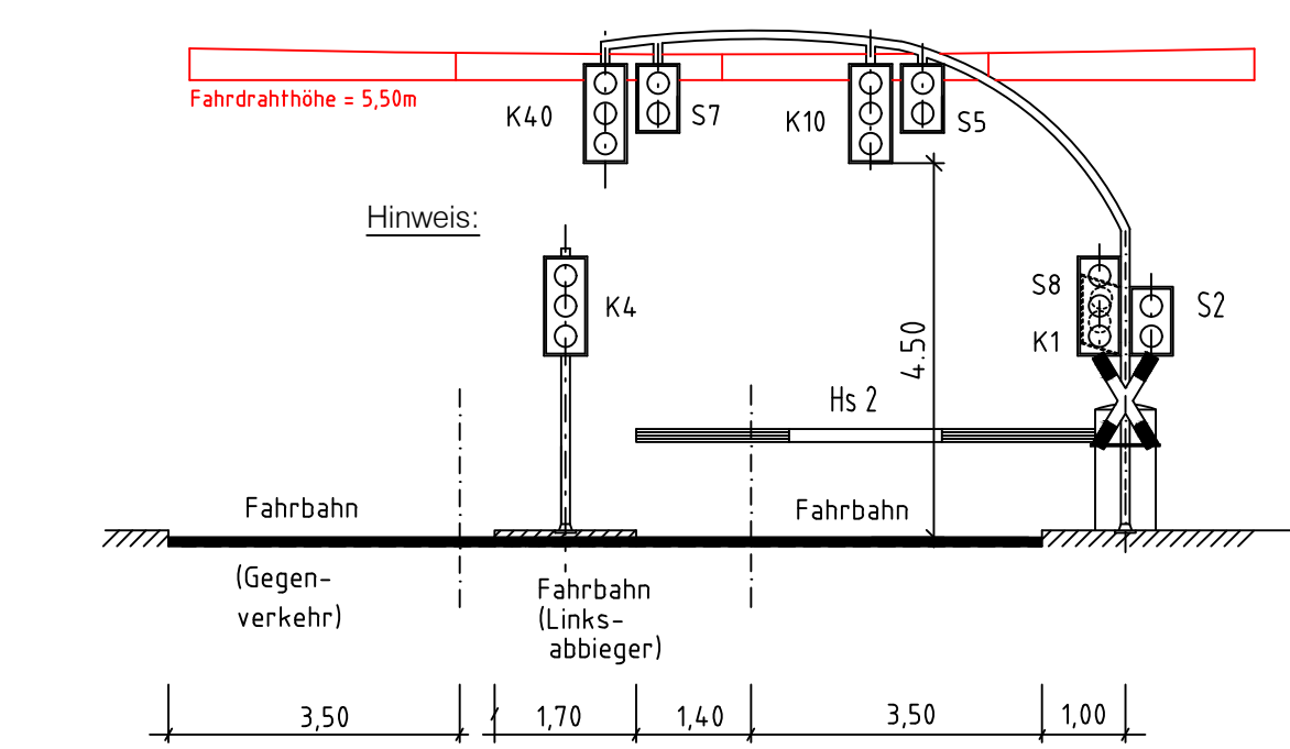
westl. Ansicht: geplante Zustand
