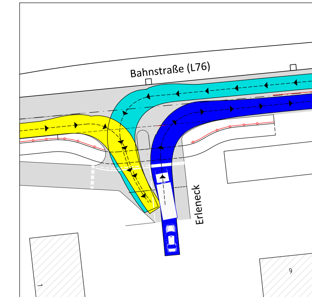
Schleppkurvenverlauf 3-achsiges Müllfahrzeug
